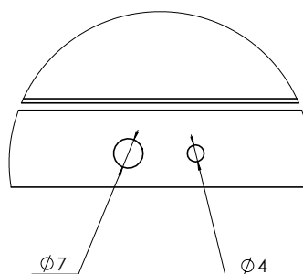
DETTAGLIO F fori per fissaggio DETAIL F holes for fixing
