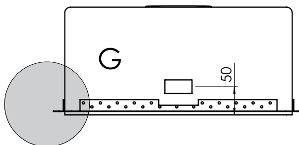
DETTAGLIO G altezza aletta per fissaggio DETAIL G wing height for the fixing
