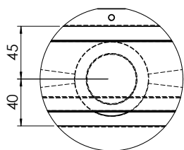
DETTAGLIO L posizione foro scarico DETAIL L drain hole position
