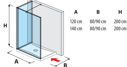
glass wall „L“ 120 x 80 cm 120, 140 x 90 cm
